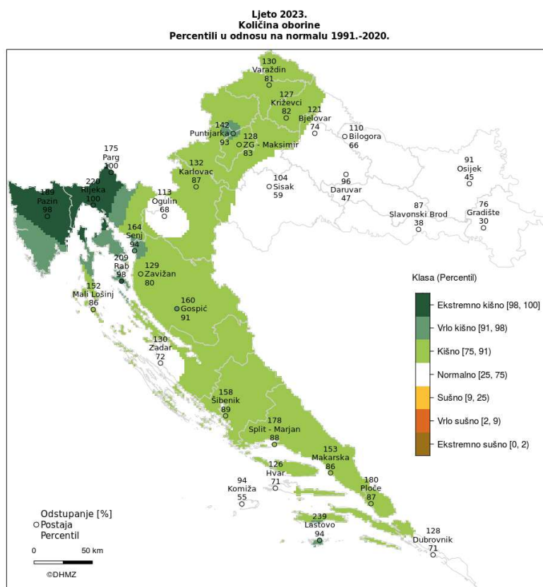
Slika 37: Odstupanje količine oborine u Hrvatskoj za ljeto 2023. godine
